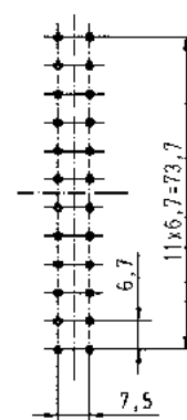
Han® 24 E
